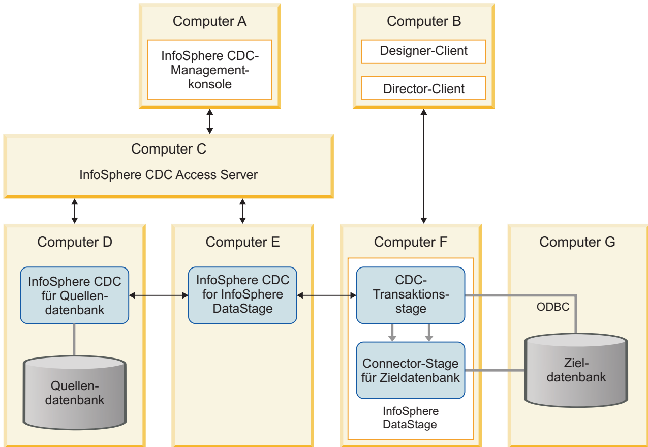
Abbildung 2. Topologie mit separaten Komponenten, die auf vielen unterschiedlichen Computern installiert sind
