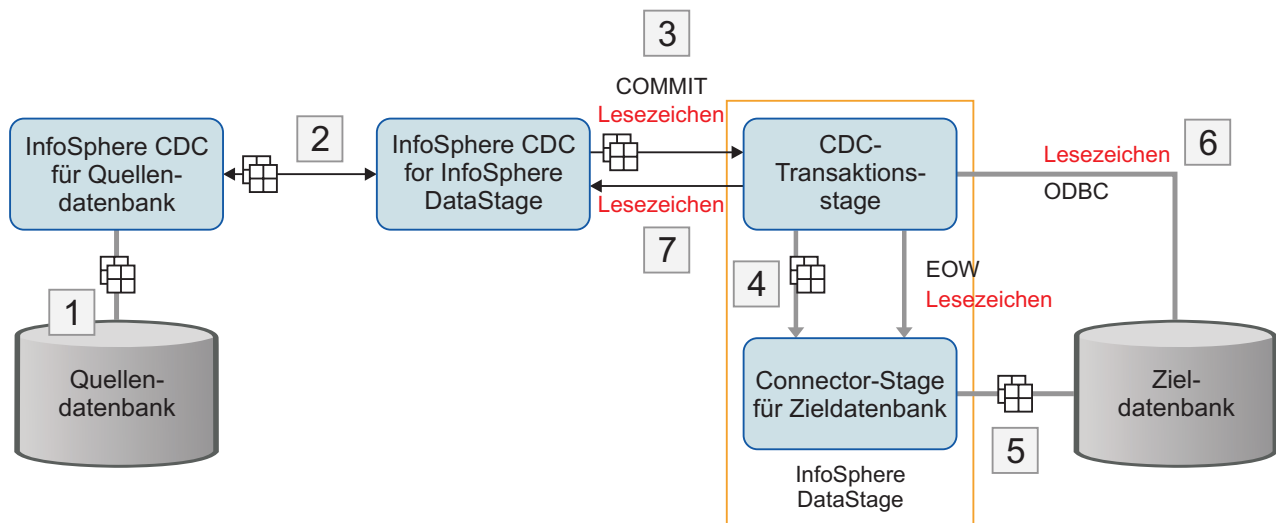
Abbildung 1. Datenfluss in einem Job der Stage 'CDC Transaction'
