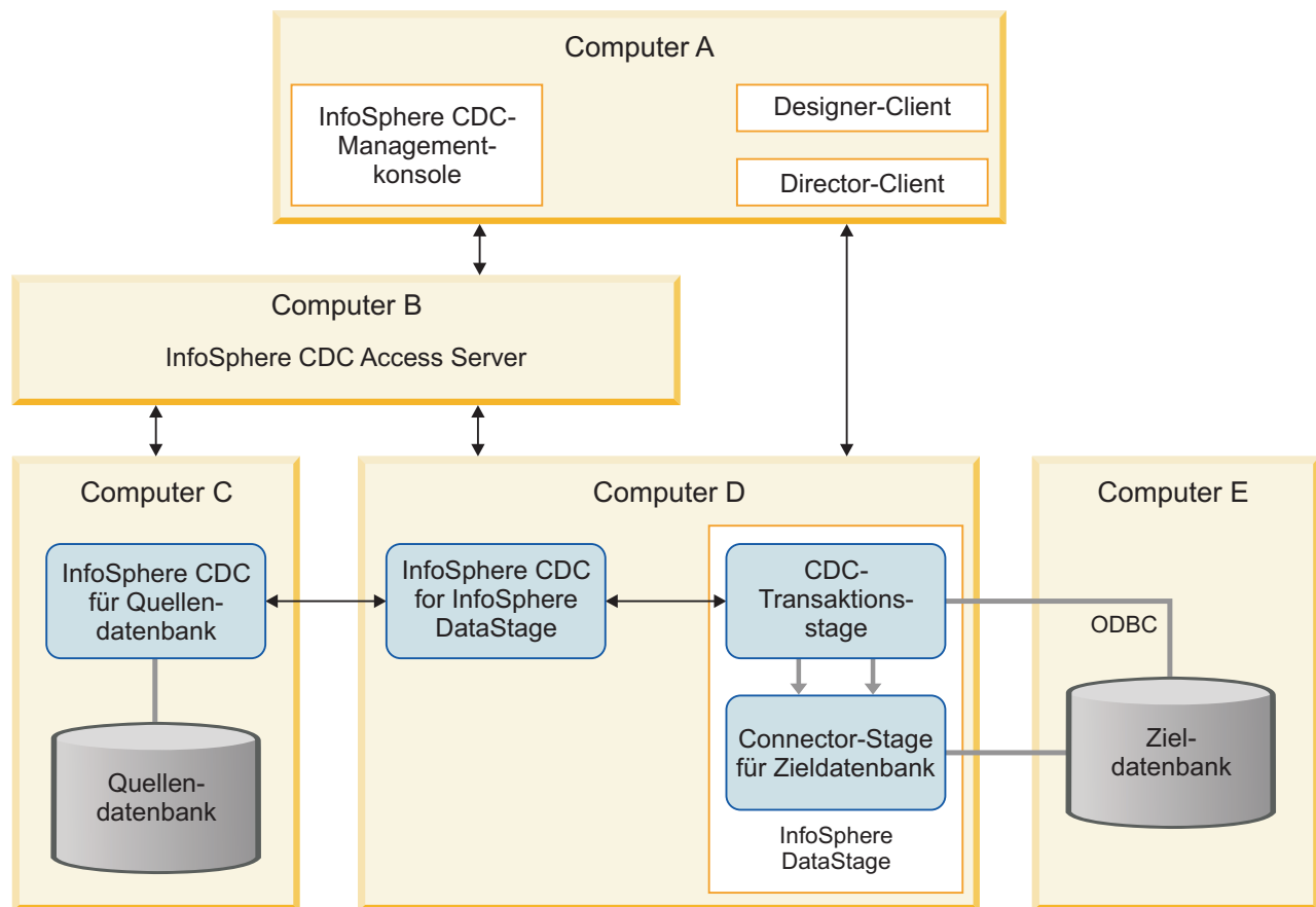
Abbildung 3. Topologie mit separaten Komponenten, die auf gemeinsam genutzten Computern installiert sind
